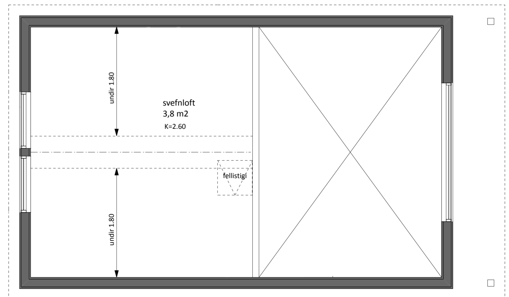
Grunnmynd svefnloft
